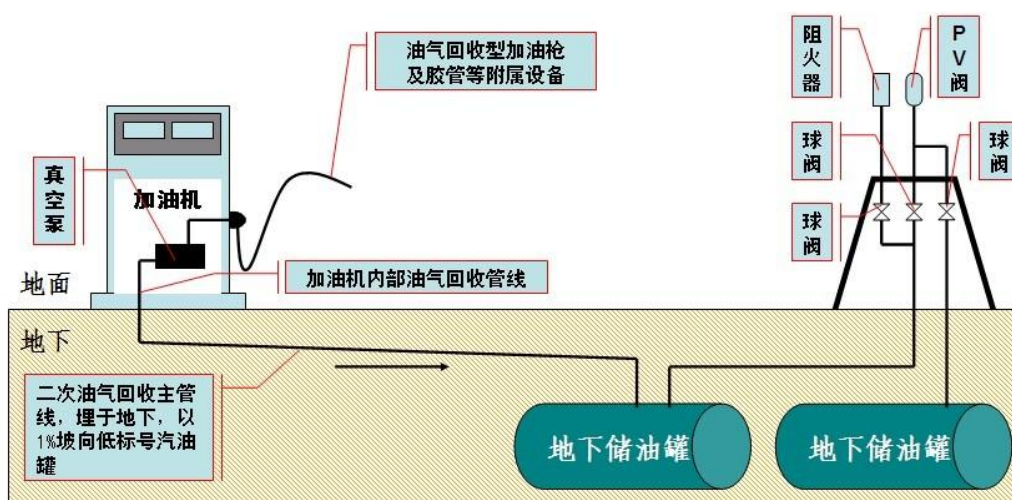
图 2-3 二次油气回收系统基本原理图
